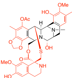
Ecteinascidin 743
