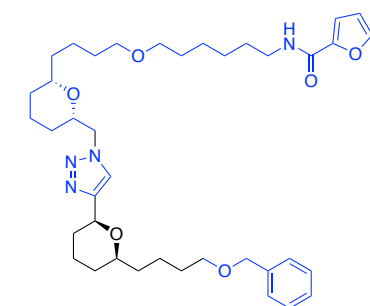
BMC 2017 , 25 , 6126.
