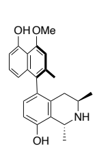
Dioncophylline C
