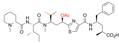
Tubulysin M
