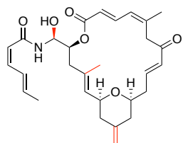
(-)-Zampanolide
