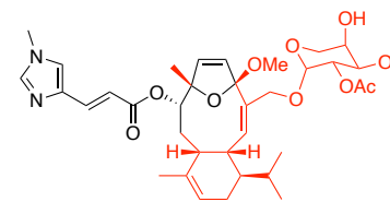
Eleutherobin
