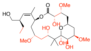
(+)-Peloruside A
