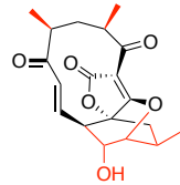
Abyssomicin C
