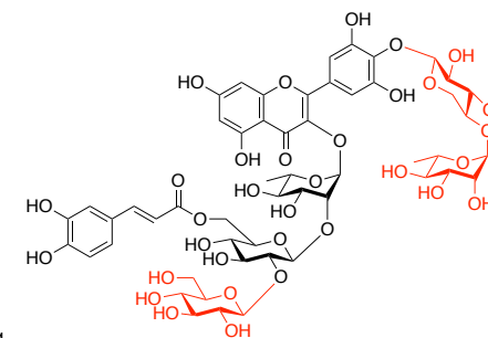
Montbretin A
