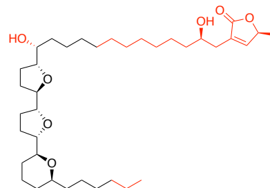
Chamuvarinin
